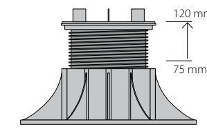
Supporto a testa autolivellante 75-120 mm 3 - 43/4 in
